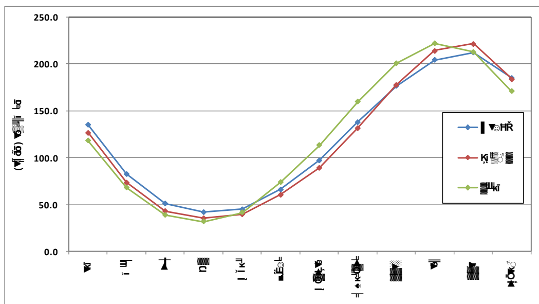
شکل ۱۶- توزیع متوسط ماهانه متوسط سالانه تبخیر از تشت در ایستگاههای منطقه (میلیمتر)
