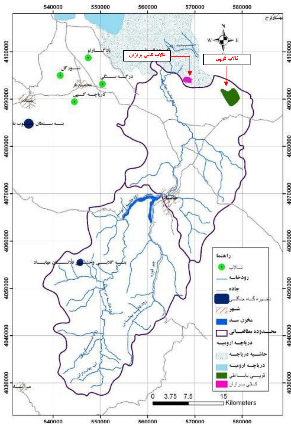
شکل ۷- موقعیت تالاب کانی برازان و حوضه آبریز مهاباد
