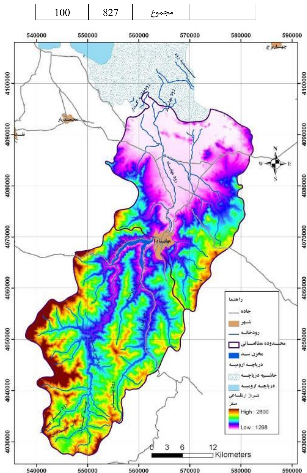
شکل ۱۸- نقشه رقومی ارتفاع محدوده مطالعاتی
